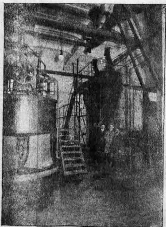
Tovarna in rafinerija špirta Petra Teslića v Sisku Aparati za mešanje in kuhanje komine.
