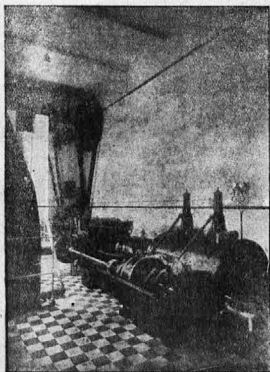
Naprava za čiščenje ječmena. Tovarna in rafinerija špirita Petra Teslića v Sisku
