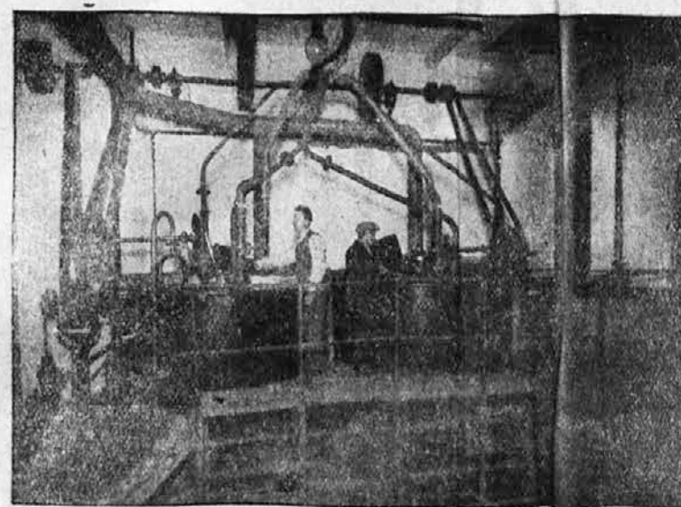
Tovarna in rafinerija špirta Petra Teslića v Sisku Aparat za mešanje komine.
