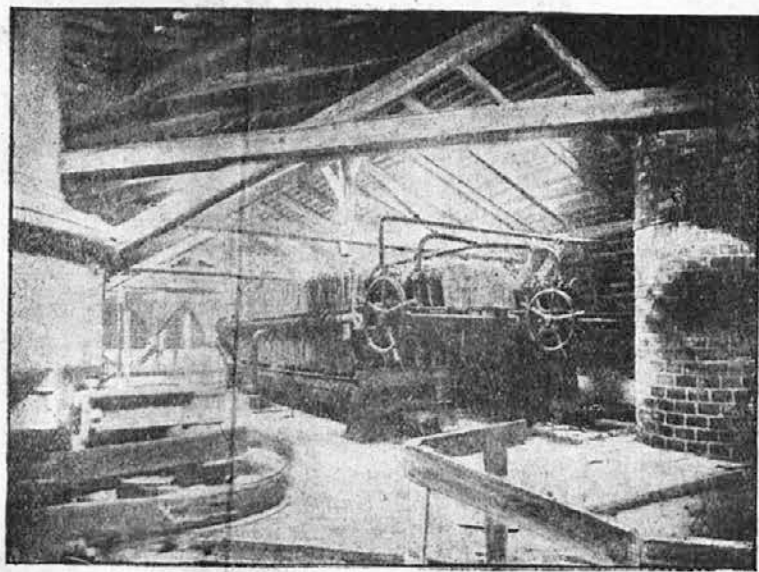
Sušilna v tovarni Petra Teslića v Sisku Aparat za prešanje mokre šlempe.
