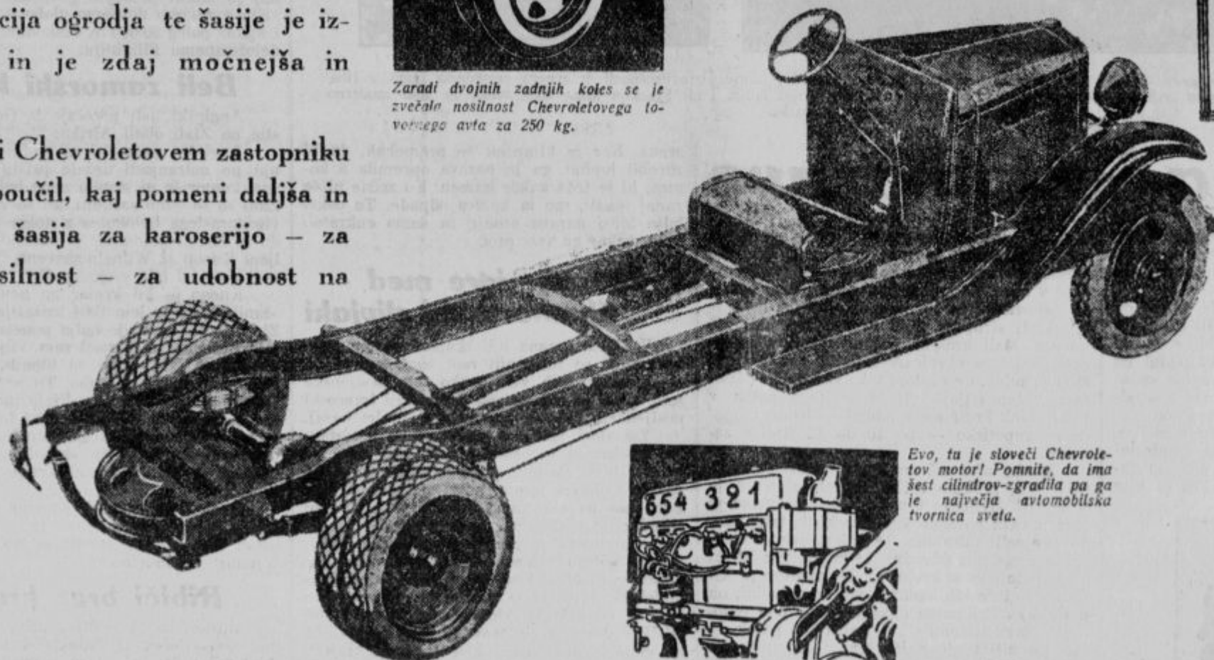
Močnejše ogradje. Ojačeno ogradje poveča odpornost Chevroletovega tovornega avtomobila — in njegova nosilnost.
