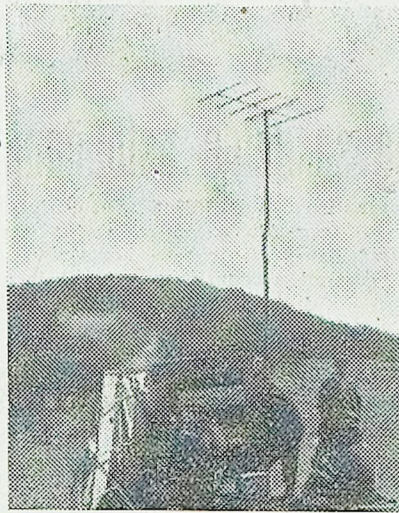
UKV ekspedicija koprskih radioamaterjev na Nanosu ob lanskoletnem evropskem UKV tekmovalstvu. Tedaj so Koprčani vzpostavili prvo UKV zvezo v razdalji nad 300 km
