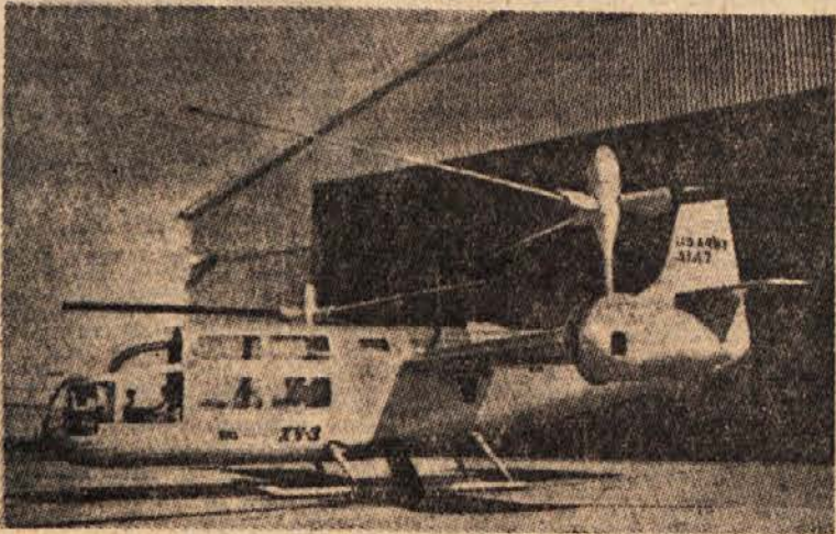
Letalo »Bell XV-3«, ki je hkrati helikopter, je dolgo 9,14 m in brez krila meri prav toliko. Motor, ki poganja oba pokončna propelerja s premerom 6,3 m, je vdelan v trupu za kabino. Hitrost znaša nad 330 km na uro.
