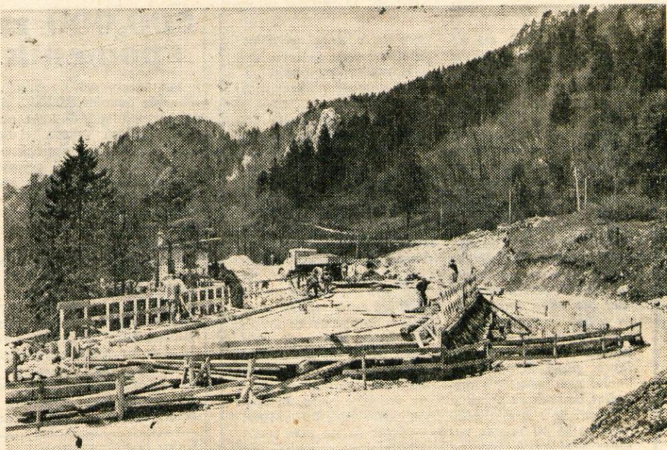
Na novem cestnem odseku Moste — Žirovnica so začeli betonirati 33 metrov dolg most čez Ratibovec. Dela opravlja splošno gradbeno podjetje Sava Jesenice. — Foto: F. Perdan
