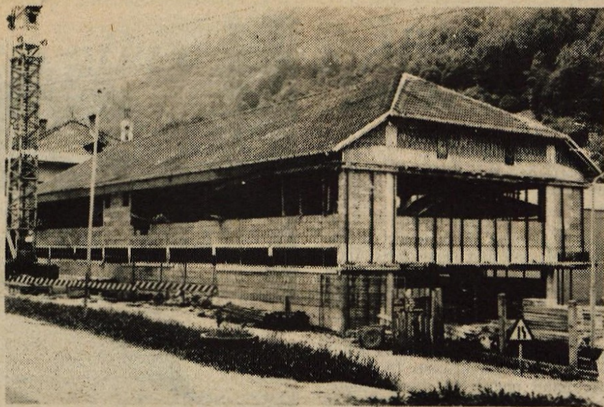
PLAMEN GRADI NOV OBJEKT - Slovenske železarne - Tovarna vijakov Plamen v Kropi gradi ob tovarni nov objekt, v katerem bodo v pritličju garaže, elektro delavnica, mehanična delavnica in mizararska delavnica. V prvem nadstropju pa bodo pisarniški prostori. Gradnja bo veljala prek 3 milijone dinarjev. - C. R. - Foto: F. Perdan
