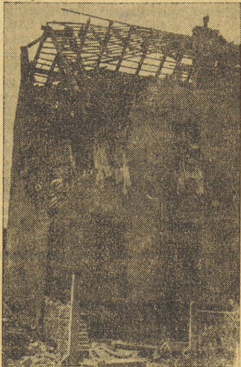
Ein durch Brandbomben zerstörtes Dach eines Wohnhauses in einem Berliner Vorort
