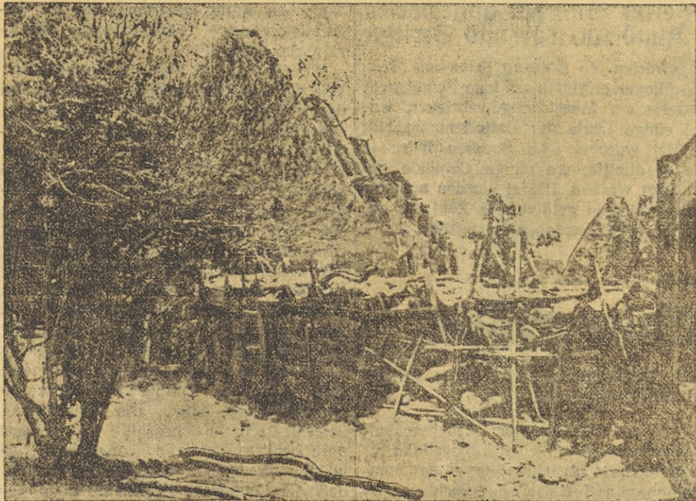
Auch im englisch-ägyptischen Sudan hatten die italienischen Truppen beachtliche Erfolge zu verzeichnen. Besonders bemerkenswert ist die Einnahme des englischen Forts Kurmuk. — Unser Bild zeigt die britischen Verteidigungsanlagen in Kurmuk nach der Erstürmung durch die Italiener
