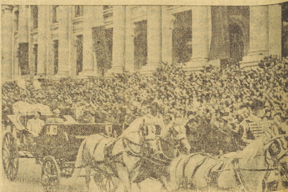
König Michael I. und seine Mutter Elena bei der Fahrt durch Bukarest
