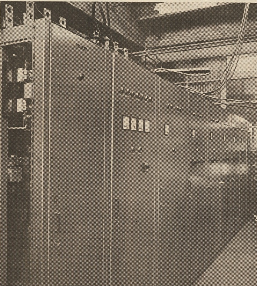
Napajalni sistem 48 V, 2400 A za mednarodno elektronsko centralo Metaconta 10 C, ki jo bo Iskra dobavila za olimpiado v Moskvi.
