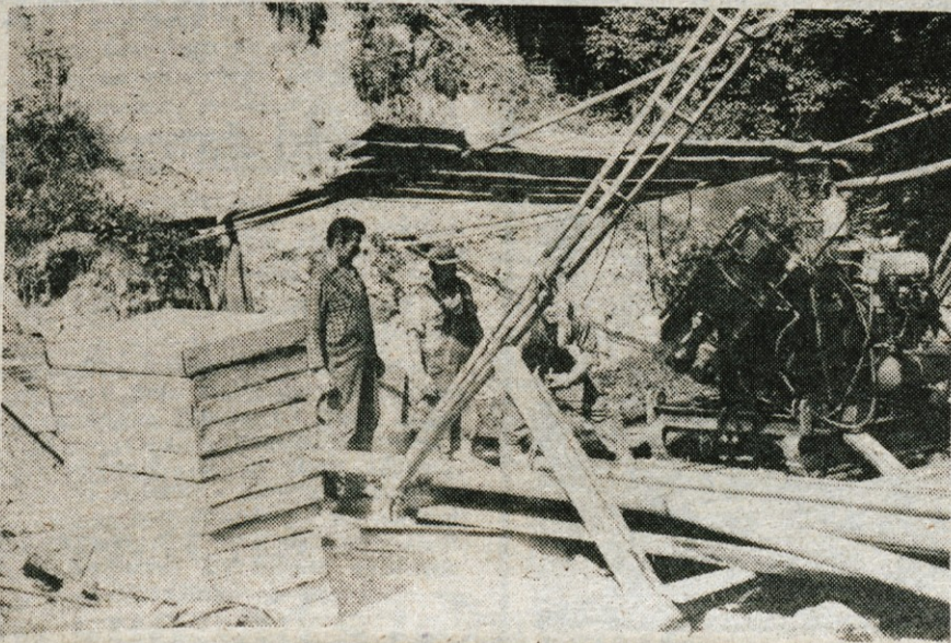
Augusta meseca so delavci Geološkega zavoda iz Ljubljane pričeli z vrtanjem v gramoznici nad Povljami (Trstenik), da bi našli nove izvirne pitne vode. Privratali so že v globino 80 m toda še vedno niso našli »pravo žilo«. Računajo, da se jim bo delo izplačalo pri 120 m, torej čez kakih 14 dni. — I. S.
