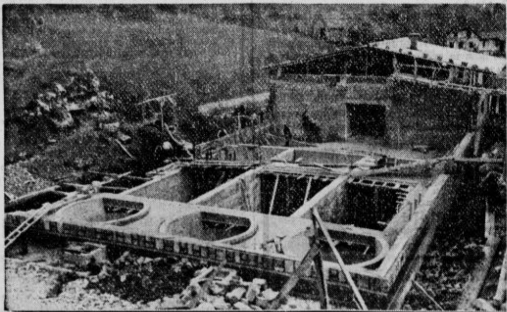
Pogled na betonirane kadunje, kamor bodo montirali čistilne naprave, ki bodo čistile in razkuževale vodo, ki bo pritekala iz zajetja v rezervoar za čisto vodo. — V ozadju stoji strojnica s črpalnimi napravami. Zgrajena je nad ogromnim podzemskim rezervoarjem za čisto vodo, ki je dolg 24 metrov, širok 10 metrov in visok 4 metre.
