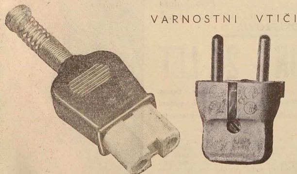
Varnostni (šuko) vtič, II-polni 10 A, 250 V
