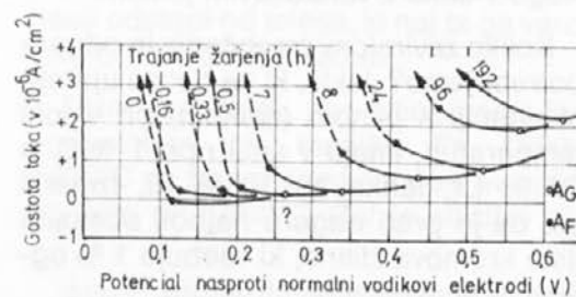
Sl. 6: Medzrnasta korozija Krivulje gostota toka – potencial v območju aktivacijskega potenciala nestabiliziranega avstenitnega jekla z 0,08 % C, 18 % Cr in 8 % Ni, katero se nahaja v 5 % vreli žveplovni kislini. Ker so vzorce jekla poprej različno žarili pri 650 °C, vidimo iz krivulj vpliv časa žarjenja na aktivacijska potenciala mej zrn (AG) in zrn samih (AF). Kot kaže, se aktivirajo (tj. izgubijo pasivnost) meje zrn pri bolj žlahtnem (večjem) potencialu kot zrna. Za oboje velja, da se aktivirajo pri bolj žlahtnem, če je čas žarjenja (izločanja karbidov po mejah) daljši.
