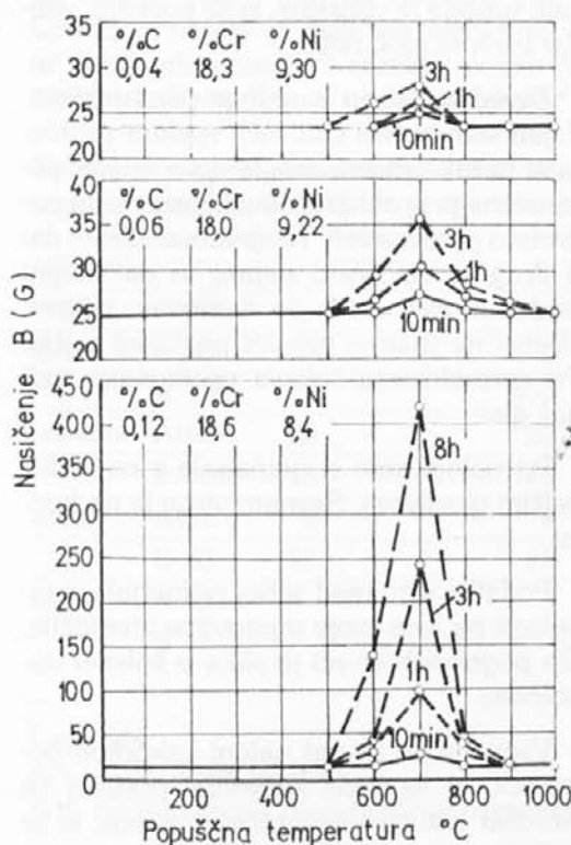
Sl. 8: Merjenje magnetnega nasičenja vzorcev iz poskusa na sliki 7 kaže nastop rahle magnetnosti – vrhovi pri popuščanju na 700^\circ\text{C} – v sicer nemagnetnem avstenitnem jeklu. Pojavil se je torej martenzit (alfa ferit). Vendar ni povzročitelj neobstoynosti jekla ta martenzit, ki ga je seveda več, če je več kroma odpotovalo iz osnove v nove karbide. Kriv je nastop ostrih skokov koncentracije kroma takoj po začetku tvorbe kromovih karbidov.
