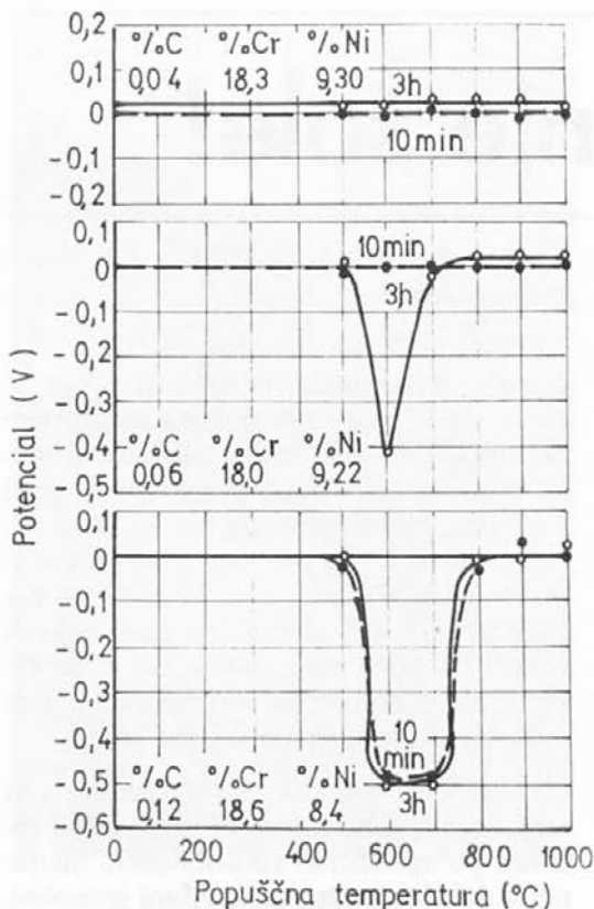
Sl. 7: Nastop neobstoynosti jekel z 18 % Cr, 8 % Ni in z različnimi vsebnostmi ogljika proti medzrnatni koroziji. Slike od zgoraj navzdol: 0,04, 0,06 in 0,12 C. Potencial nasproti vodikovi so merili v 1n – žveplovni kislini. Preizkušance so poprej žarili bodisi 10 minut bodisi 3 ure pri kateri od temperatur, prikazanih na vodoravni osi diagrama. Vidimo, da pasivnost – ki je v taki kisli raztopini pri OV – popusti jeklu z 0,06 % šele po 3 urah žarjenja, jeklu z 0,12 % pa že tudi po 10 minutah. Če dolgo – 20 dni – žarimo kje pri 550 – 700°C jeklo, ki ima celo komaj 0,01 % C, mu tudi pade potencial in se začne razpad – ločevanje zrn.
