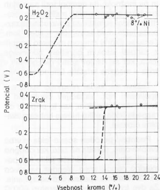
Sl. 3: Vsebnost kroma, ki že daje pasivnost jeklu je, močno odvisna od oksidacijskega potenciala korozijskega okolja.
