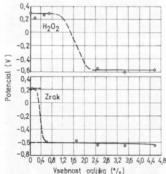
Sl. 4: Vpliv ogljika na potencial kromovega jekla v žvepleni kislini. Krivulji kažeta, da od začetne pasivnosti jekla s 14 % Cr in nič ogljika prehaja do aktivnosti jekla, če je v njem poleg 14 % Cr že 0,1 % C in je v okolju zrak. Če je ob elektrodi H 2 O 2 , sme biti le-ta iz jekla z desetkrat več ogljika, pa bo še zmerom pasivna (obstoja proti koroziji).
