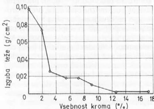
Sl. 1: Že majhni dodatki kroma jeklu izboljšajo obstojnost proti koroziji v industrijskem zraku. Nad 13 % Cr pa ni treba.
