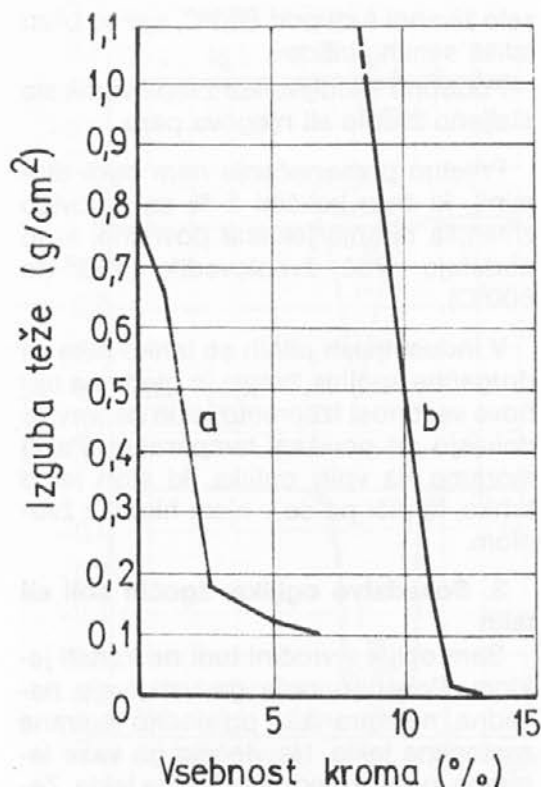
Sl. 2: Izgube teže izdelkov z različnimi vsebnostmi kroma so merili po 30 dneh v žveplasti kislini (21 C) ali v 5 % solitni kislini.
