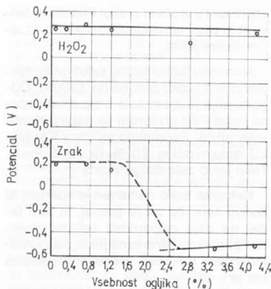
Sl. 5: Vpliv ogljika na potencial jekla z 20 % Cr in 8 % Ni v žvepleni kislini, ki ji dodajamo bodisi zrak bodisi H 2 O 2 . V tem drugem primeru je jeklova pasivnost neuničljiva, neodvisna od vsebnosti ogljika v njem, kot kaže zgornja vodoravna črta.
