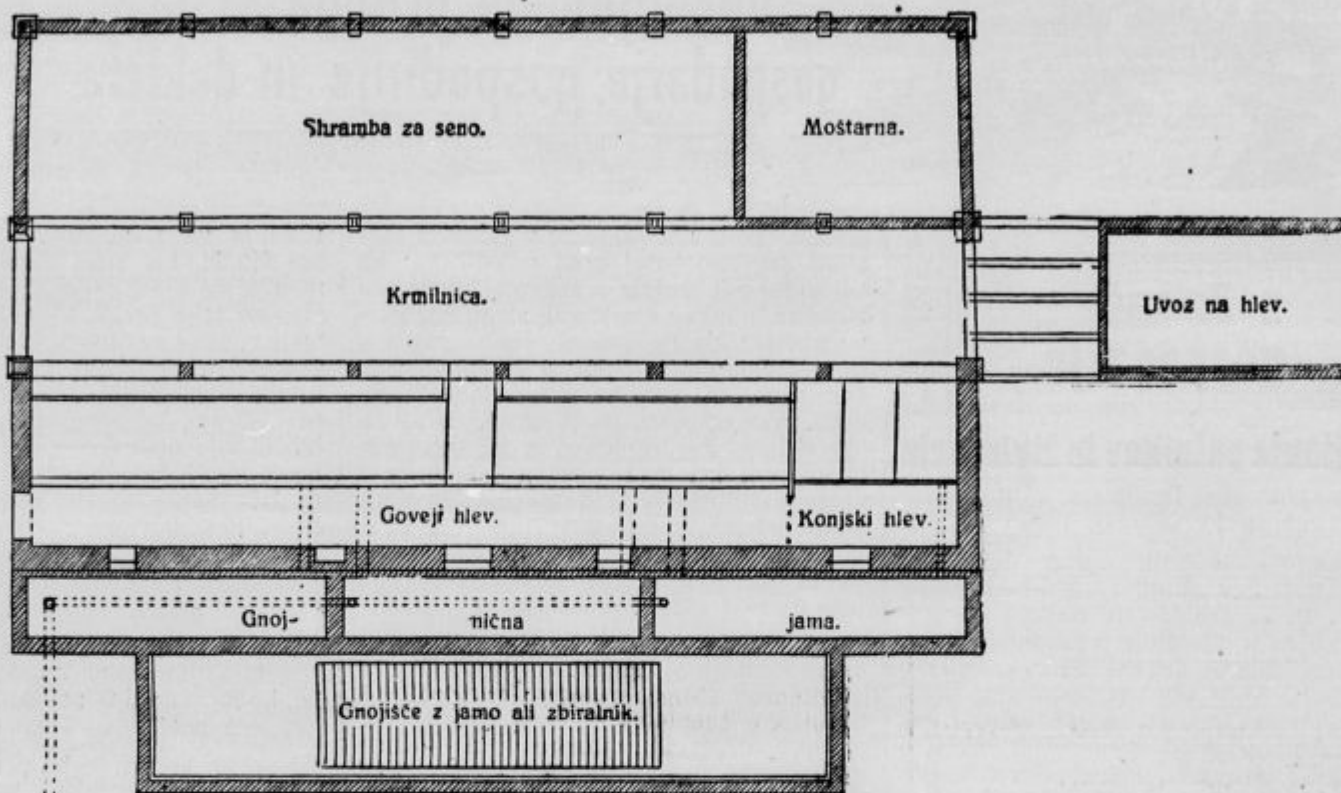
Prerez hleva in gnojišča.
