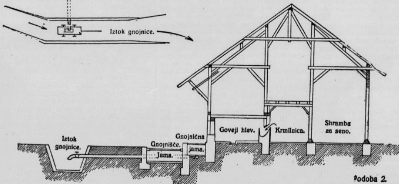
Prerez hleva in gnojišča.
