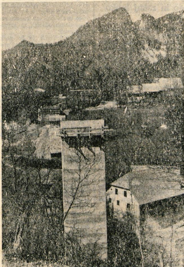
Dvema stebroma novega mostu čez Završnico se bo v kratkem pridružil še tretji in zadnji steber. Nov most bo dolg 142 metrov in bo kombinacija železnih nosilcev z betonsko ploščo. foto: F. Perdan
