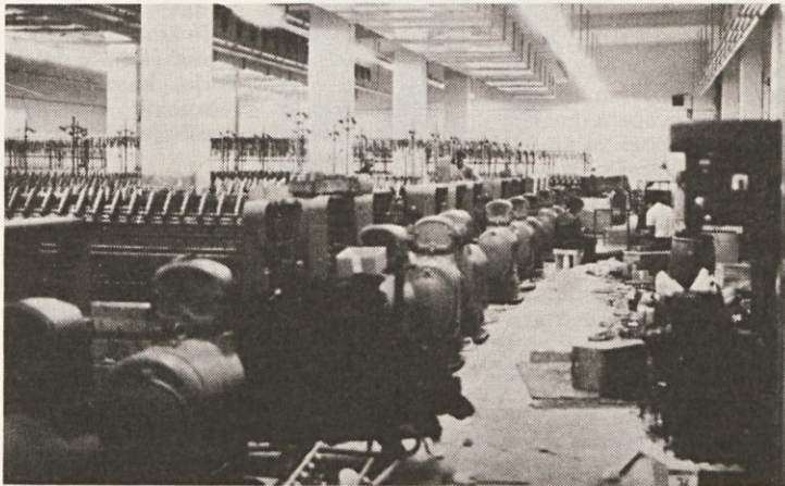
V prizidku predilnice v 2. nadstropju renovirani stroji še niso povsem zmontirani.
