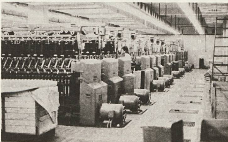
Stroji v prizidku predilnice v 1. nadstropju
