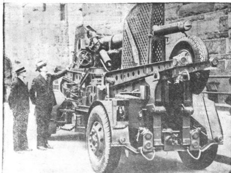
AMERISKI TOPOVI PROTI LETALOM. V Bostonu, Massachusetts, so nedavno kazali ljudem protiletalski top, ki lahko izstrelji vsako minuto 25 nabojev do višine 9000 m
