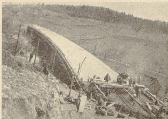
Gradnja avtomobilske ceste Ljubljana—Zagreb. 148 m dolgi viadukt pri Stični med gradnjo. Nova avtomobilska cesta bo speljana ob desnem bregu Krke
