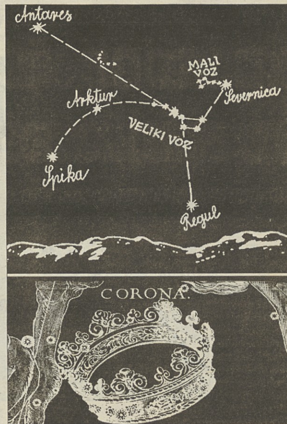
Zgoraj: Takole po Velikem vozu najdemo ozvezdja Severna krona, ki je vidno zvečer od marca do oktobra. Glavna zvezda ozvezdja je Dragulj (Gemma). Spodaj: Silka Krone iz starejšega zvezdnega atlasa
