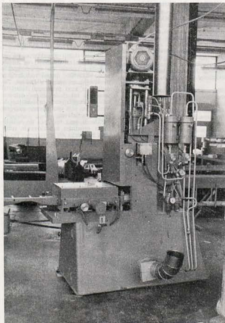
Krožna žaga za koničenje elementov — lastne konstrukcije.
