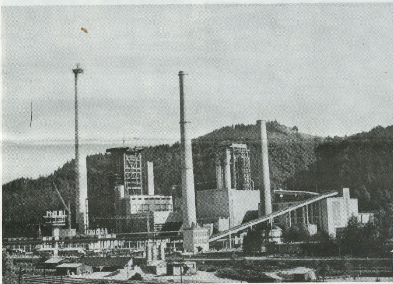
Naša elektrarna, od desne proti levi — I. faza (2 x 30 MW) in II. faza (1 x 75 MW), III. faza (1 x 275 MW) ter TEŠ IV (1 x 335 MW) v izgradnji
