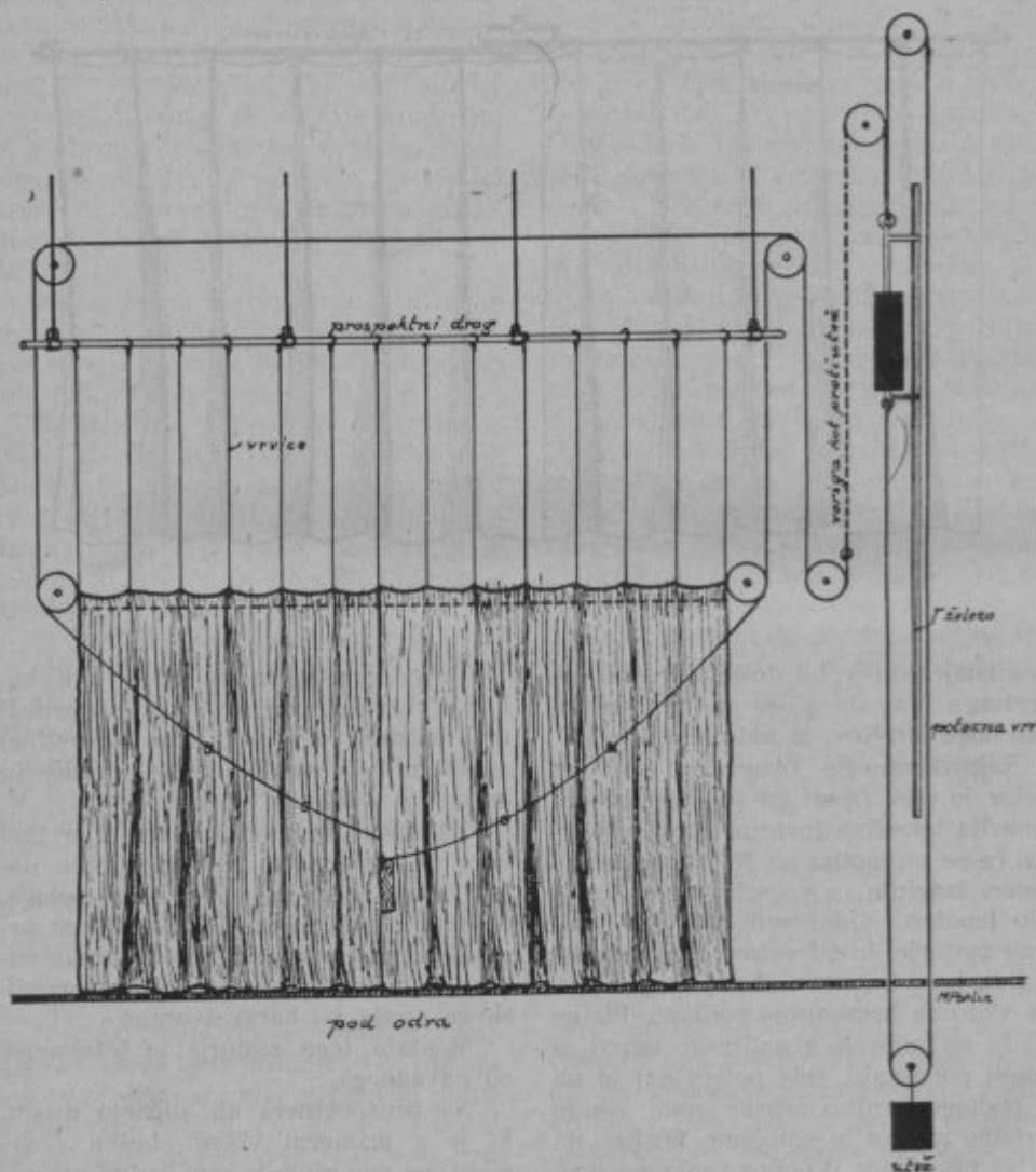
Francoški zastor (zaprt).
