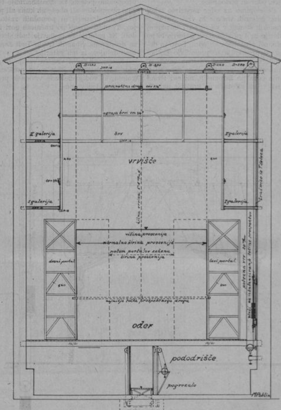
Prerez odra.
