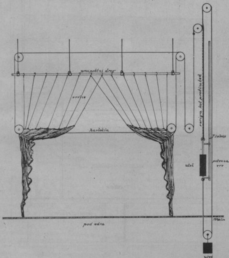
Francoski zastor (odprt).
