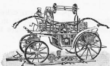
Štirikolesne vozne brizgalnice. Konopne in lanene cevi lastnega izdelka, surove in gumirane. Gumaste špiralne cevi, navijaki, sklopniki, mlaznice, razpr- ševalniki Pomočki za popravljanje cevi.
