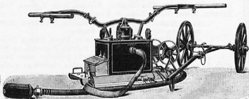
Dvokolesne snemalne brizgalnice z vodohranom ali brez njega, na ročni kolnici ali za konjsko vprego.
