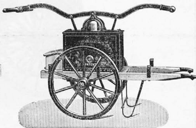
Omaraste brizge s premakljivo osjo.
