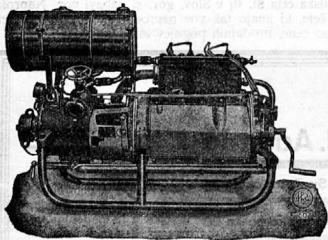
Dvocilindrska motorna brizgalnica, model 1929, 18/20 HP., pritisk do 16 atmosfer. Hladilnik novega sistema, ogrevanje črpalke s toplo čisto vodo.
