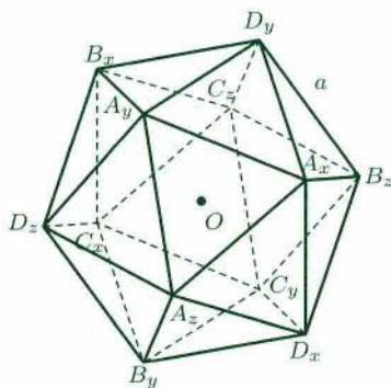
Slika 4. Pravilni ikozaeder.
