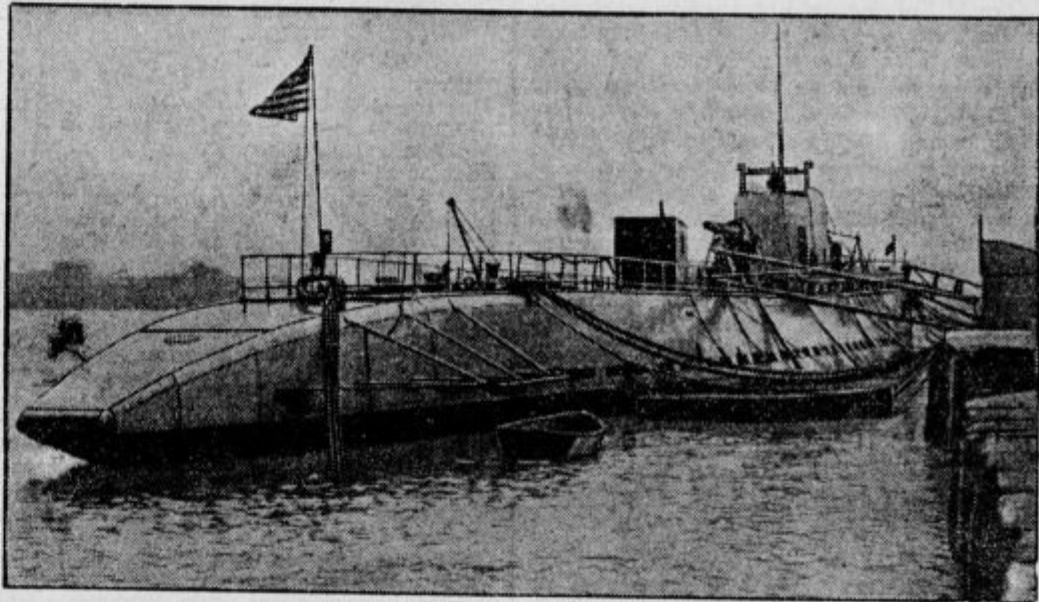
Največja podmornica sveta. Združene države v Ameriki so zgradile ogromno podmornico »V 5«, ki je opremljena z najmodernejšimi varnostnimi in strelnimi pripravami. V najkrajšem času bo podmornica v San Diego odplula na svojo prvo poskušno vožnjo.
