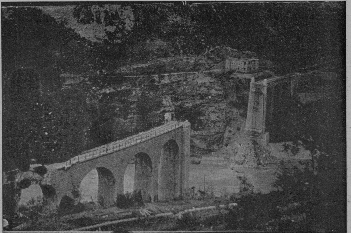
Ostanki krasnega železniškega solkanskega mostu pri Gorici, ki je bil eden največjih mostov na svetu.
