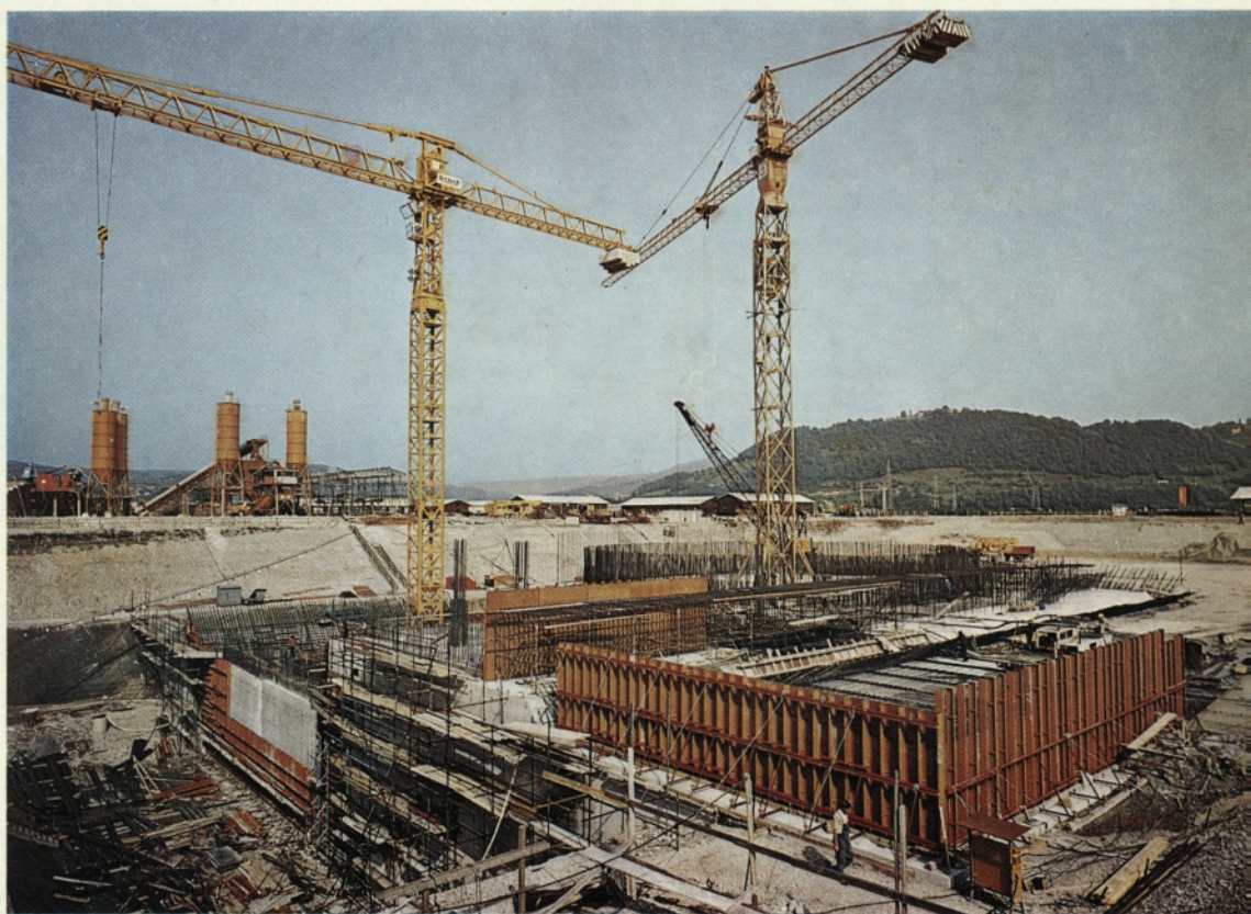
Izgradnja prve jedrske elektrarne v Jugoslaviji Izvajalec GIP GRADIS (Foto: Exportprojekt)
