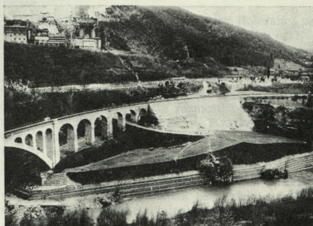
Sl. 14. Pogled na levi breg po sanaciji
