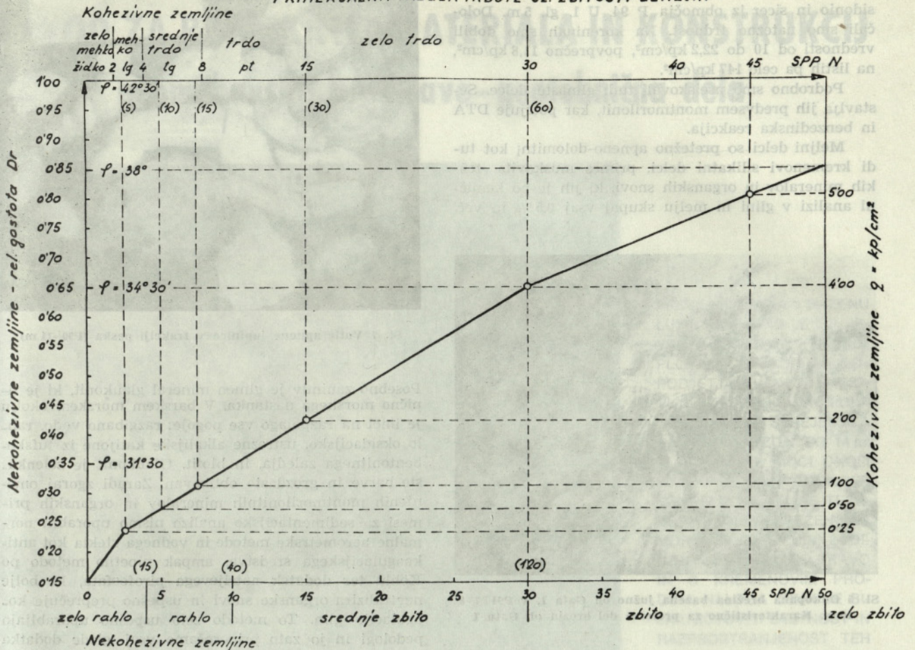
Sl. 2 Diagram gostote D_r pri nekohezivnih ter trdnosti ( q ) kohezivnih zemljin v primerjavi s standardno penetracijo
