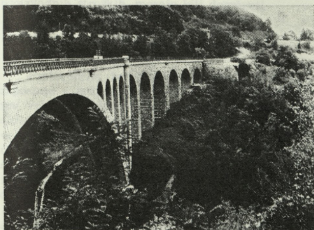
Sl. 13. Pogled na levi breg pred sanacijo
