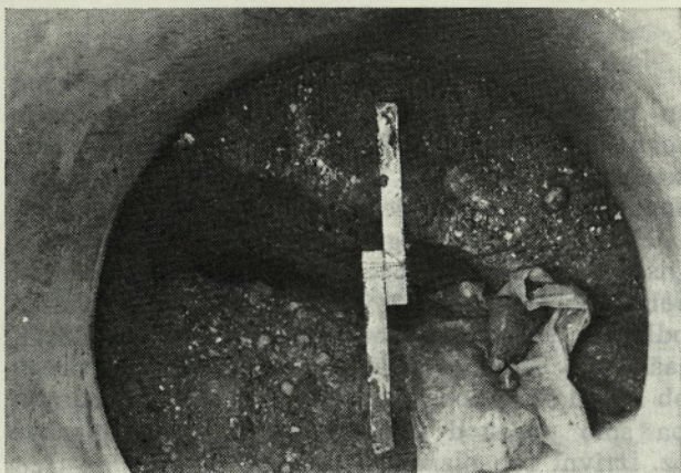
Sl. 3. Razpoka v konglomeratu na mestu jaška J 8
