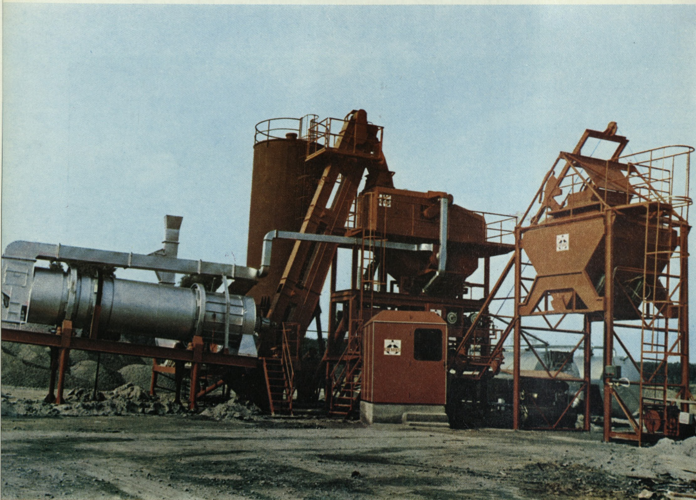
Asfaltna baza AB 4-40 proizvodnje Gradis — TOZD KO MARIBOR
