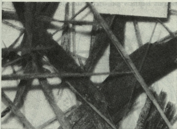
Sl. 6 Mikroskopski posnetek ostankov morskega rastlinstva v frakciji peska (P90/-11 m)
