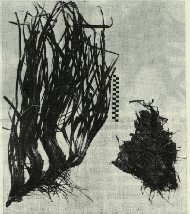
Sl. 4 Vzorci Trave » Posidonia oceanica « iz Bara, sveža na površini (levo), in korenine v bazenu ob Gatju I (P94/-5 m)
