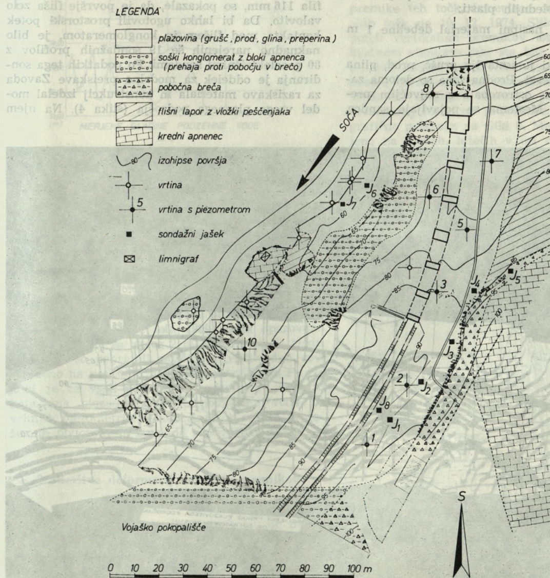
SI. 2 MOST NA SOČI - SITUACIJA
