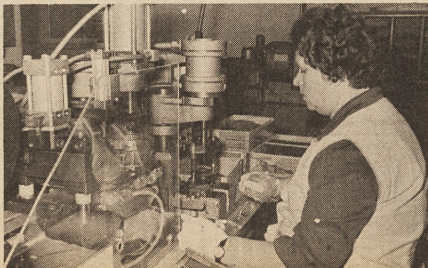
Jožica Sargo pri oblikovanju membran iz makrofol folije za telefonski vložek SL-5.
