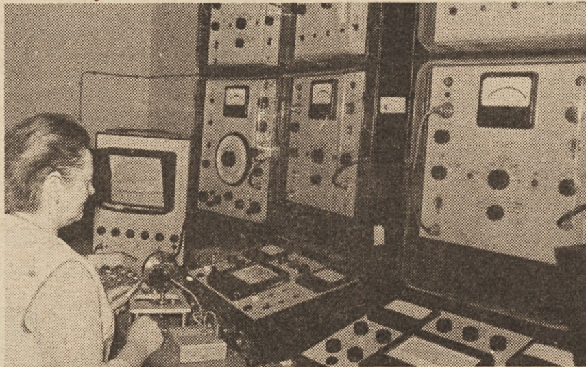
Stefka Kavaš meri občutljivost mikrofonskega in telefonskega vložka.
