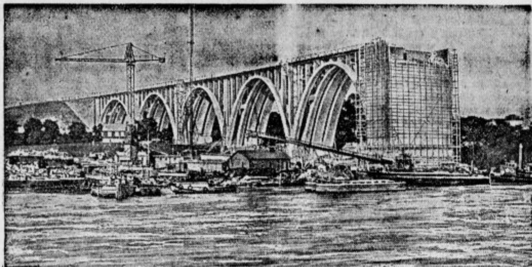
Pogled na prvi betonski opornik ob Jutlanski obali za železobetonski most iz petih velikanskih lokov, ki veže prvi opornik v morju z jutlansko celino. Ob mostu je nastala prava kolonija in ladje, ki jih vidimo na sliki, so vse pomagale pri graditvi.
