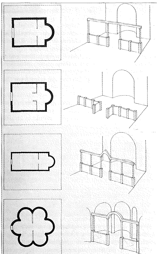
Sl. 6: Rekonstrukcija različnih oblik kornih pregraj v zgodnesrednjeveških hrvaških cerkvicah (rekonstrukcija povzeta po Rapanić, 1987).
