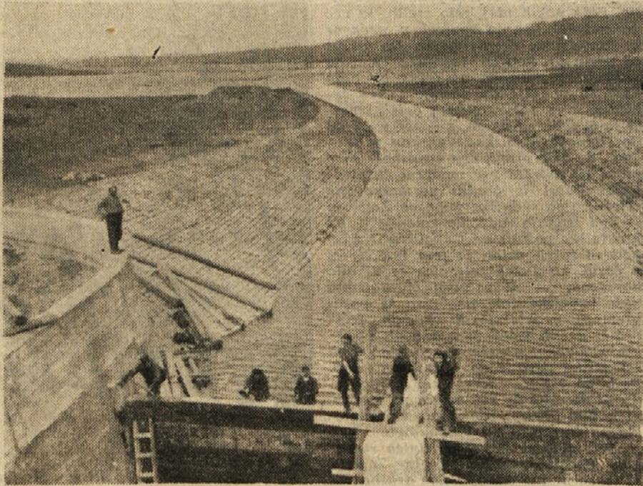
Vlasinsko jezero z odločnim kanalom za hidrocentralo
