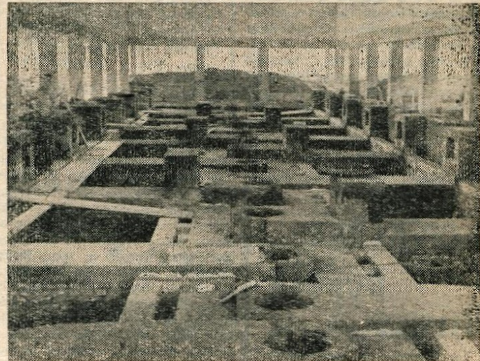
V opekarni Češnjek bodo kmalu dograjene nove peči
