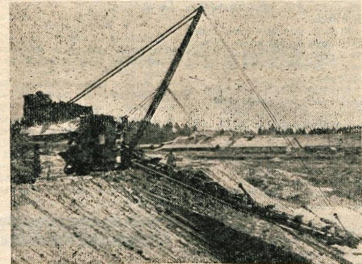
Izkop ilovice v opekarni Bobovk
