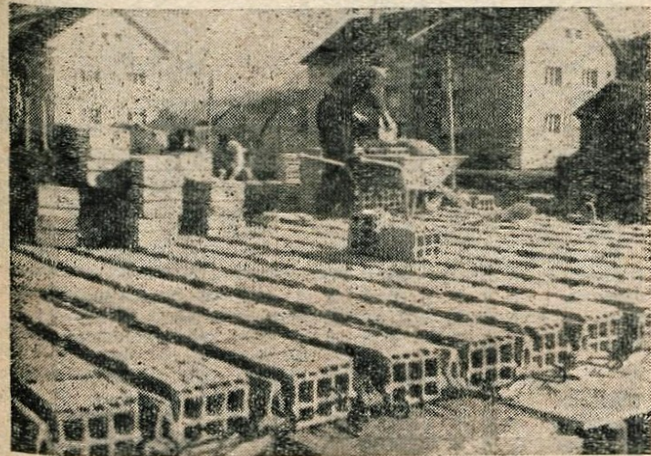
Montažni strop »RAPID« iz opečnih izdelkov — Gradnja stanovanjskih blokov v Skofji Loki
