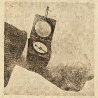
Tudi ročni kompas »M. 52« je eden od izdelkov te tovarne, ki ga pri nas prvi izdelujejo. Namenjen bo rezervnim oficirjem, planincem, turistom - komurkoli. S kompasom, in zlasti če ima še zemljevid, se bo vsakdo lahko znašel in krenil v pravo smer iz samotnih krajev, in je in drugih ovir, ki so v takih krajih lahko usodne.
