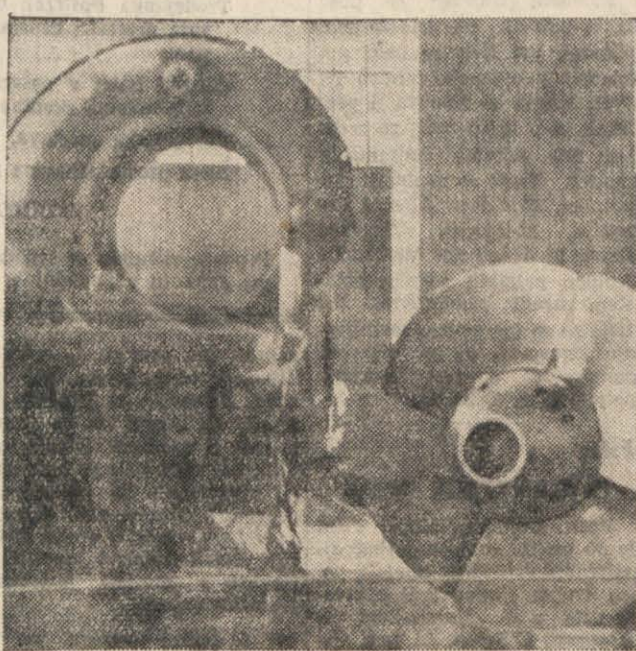
Na zagrebskem velesejmu vzbujajo veliko pozornost izdelki Titovih zavodov «Litostroj» v Ljubljani. Na sliki vidimo v ospredju na levi strani Kaplanovo turbino (2.200 konjskih sil) za hidrocentrale Sokolovica na Timoku v Srbiji s pripadajočim propelerjem na desni strani. V ozadju pa je postavljen orjaško ohišje Franciscove turbine za hidrocentrale Moste pri Zirovnici, ki bo imela 7.500 konjskih sil.
