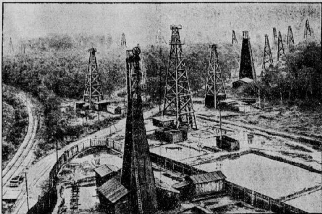
Nova najdišča petroleja na Hanoveranskem. Vrtalni stolpi na petrolejskem ozemlju. Na Hanoveranskem so odkrili nov, znaten studenec petroleja, na kakršnega doslej v Nemčiji še niso nalezli. Vsako uro priteče do 16 ton petroleja.
