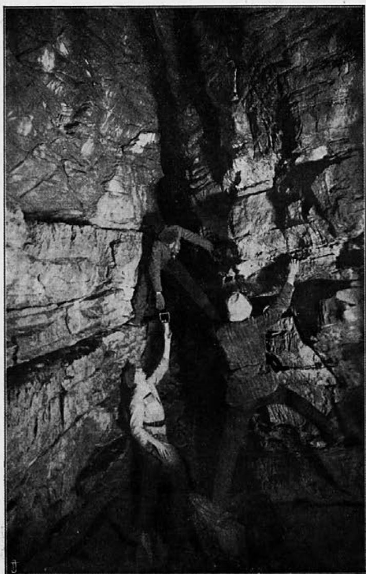
Široka jama pri Glažuti pod Veliko goro pri Kočevju. (K članku: Podzemski svet.)
