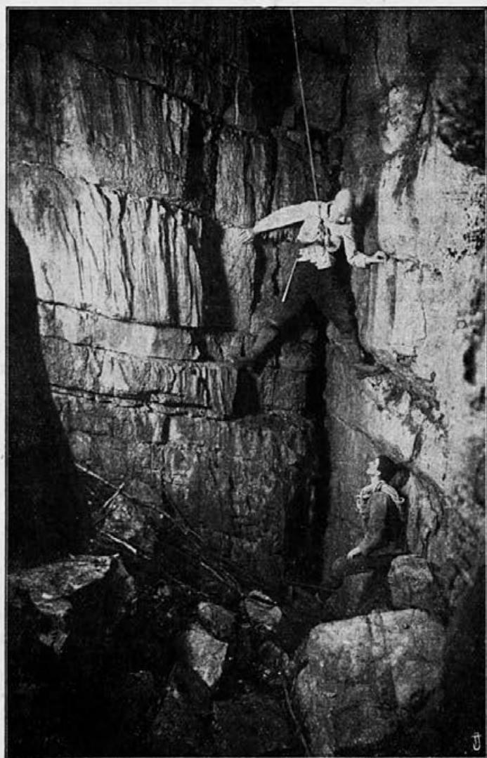
Žlebičaste stene v Mačkovi jami nad Podpečjo v Dobropoljah. (K članku: Podzemski svet.) .....
