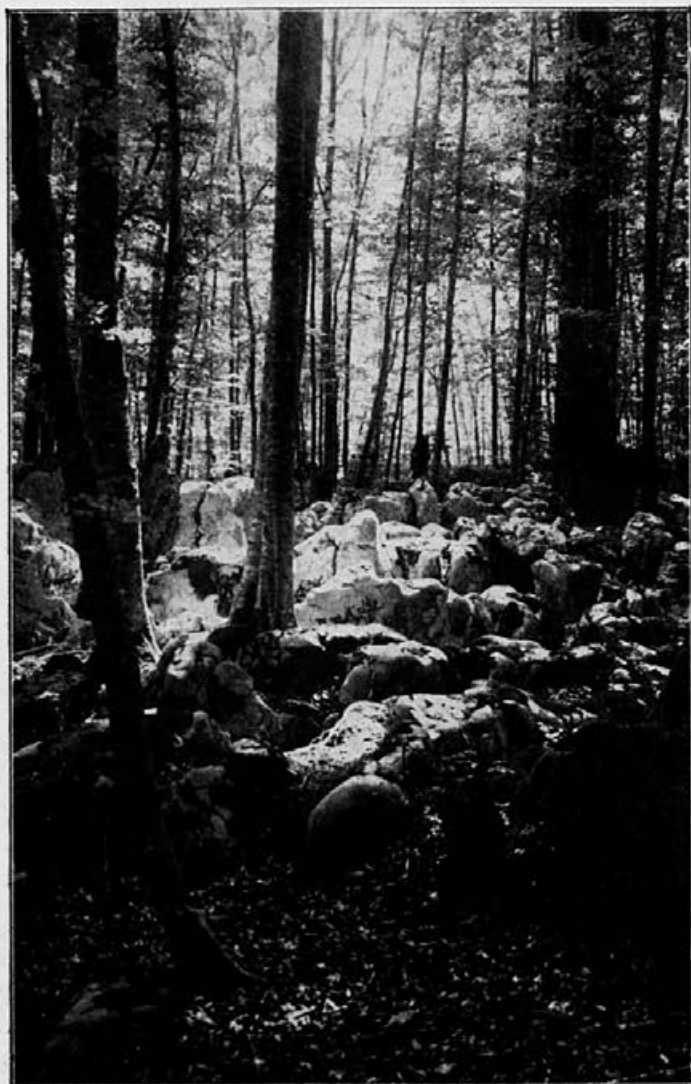
Žlebovje v Kraškem gozdu.
