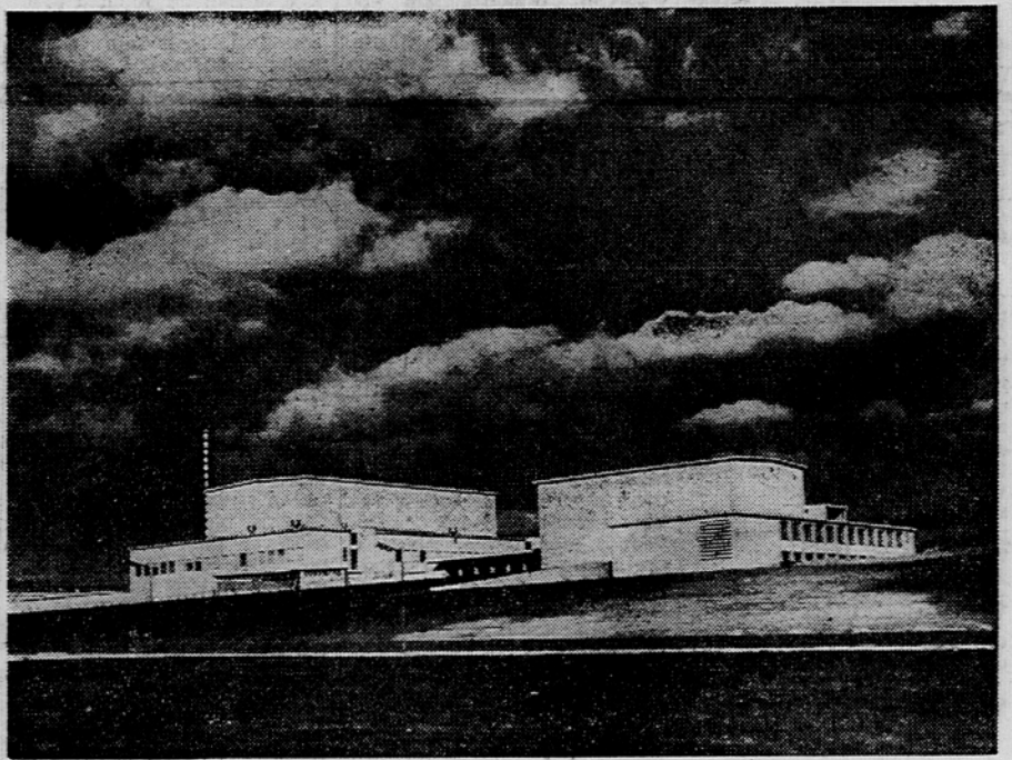
Zgradba velikega reaktorja v Vinči
