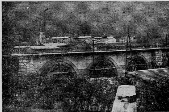
Železniški most v Hrastniku so obnovili mesec dni pred rokom. Pri obnavljanju in razširjanju mostu so izkopali precejšnje količine zemlje in porabili precej gradbenega materiala. V ozadju slike je novo steklarsko naselje na Savi.
