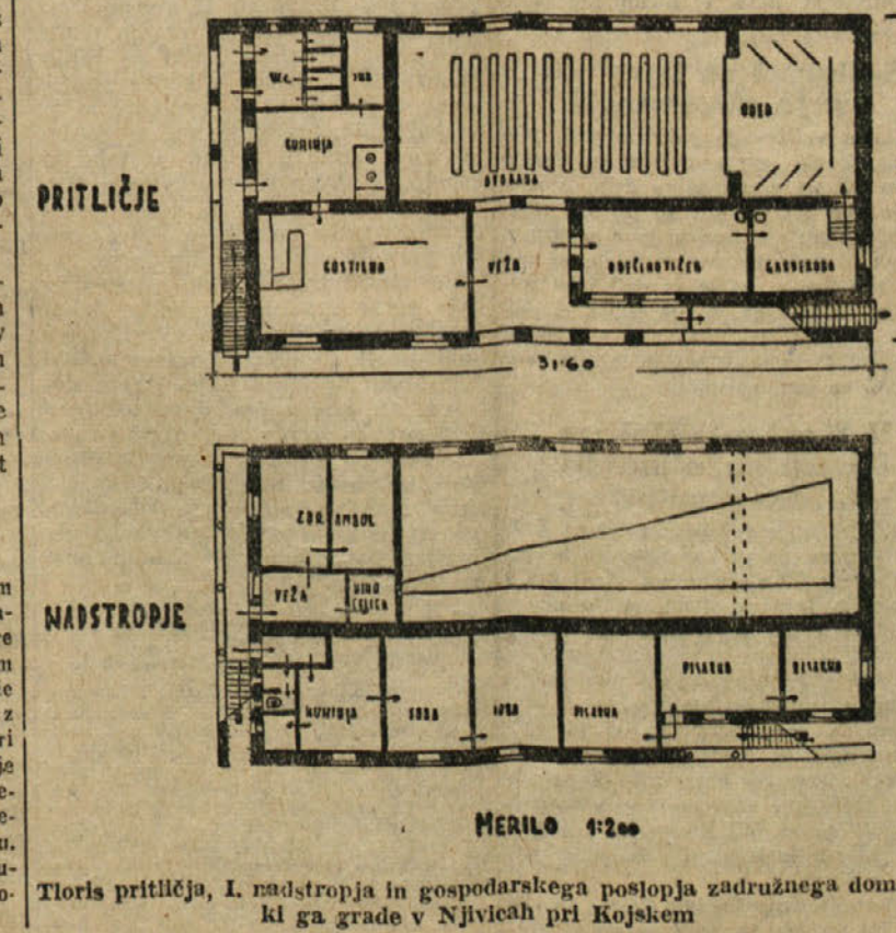
Tloris pritličja, I. nadstropja in gospodarskega poslopja združnega doma, ki ga grade v Njivicah pri Kojsem
