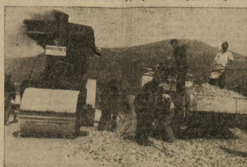
Težek parni valjar utrjuje cestnice glavne magistrale v Novi Gorici. Mladinske brigade tekmujejo, da bi gradnjo čim bolj pospešile
