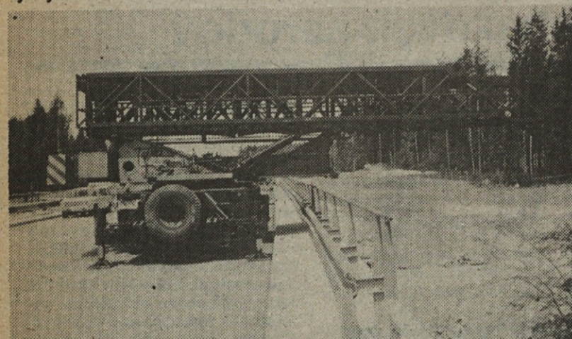
Zavrtitev nadgradnje za 90° v horizontalni ravni
