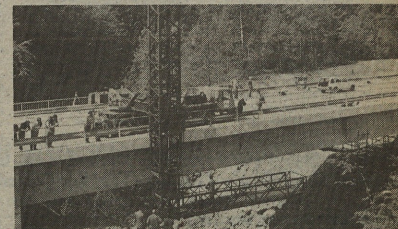
Delovni hodnik zasukan za 90°, teleskopski del stolpa izvlečen na potrebno višino
