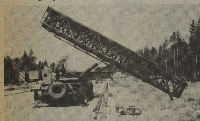
Nagibanje nadgradnje v vertikalni položaj
