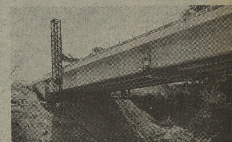
Hodnik zasukan pod most — delovni položaj naprave
