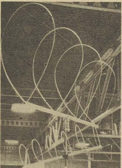
Domača konstrukcija antene za UKV zveze delta Loop YU 3RM na razstavi izdelkov radioamaterjev
