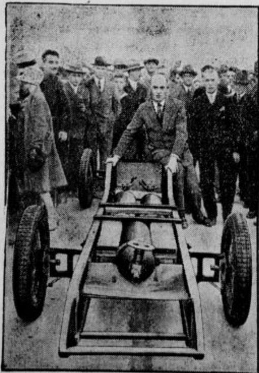
Novo vrsto avtomobil. Pri Essenu preizkuša Valier svoj novi voz, ki ga poganja stisnjen zrak in ki je brez nevarnosti za voznika in gledalca.
