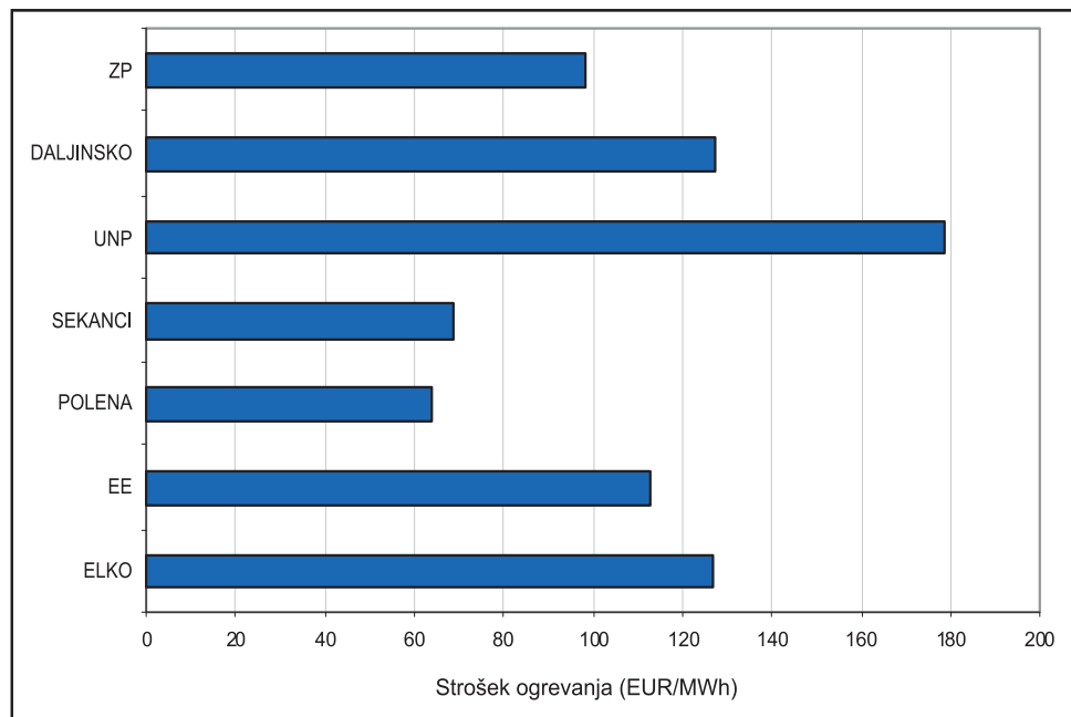
Graf 1: Celoten strošek ogrevanja povprečne enodružinske hiše, Ptuj, september 2008
