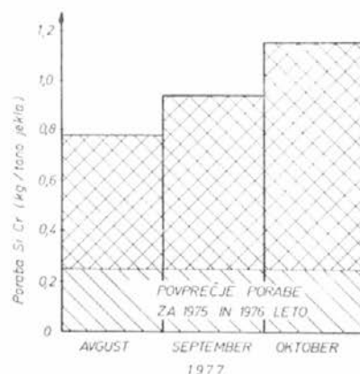
Slika 7: Povečanje porabe Si Cr na tono izdelanega jekla
