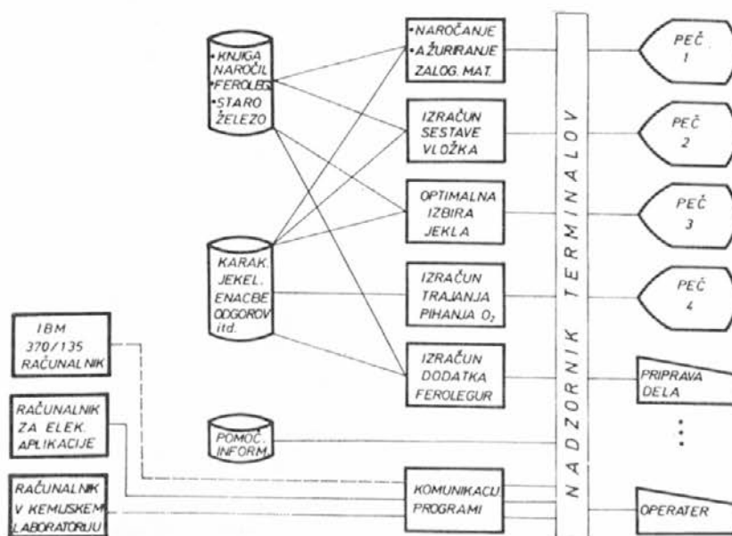
Slika 2: V Železarni Ravni uporabljeni AVTOMET programi
