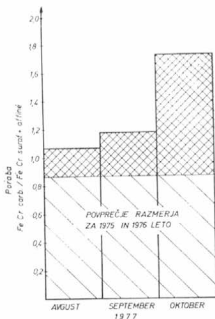
Slika 8: Povečanje porabe Fe Cr carburé v primerjavi s porabo Fe Cr surfactin in aff.
