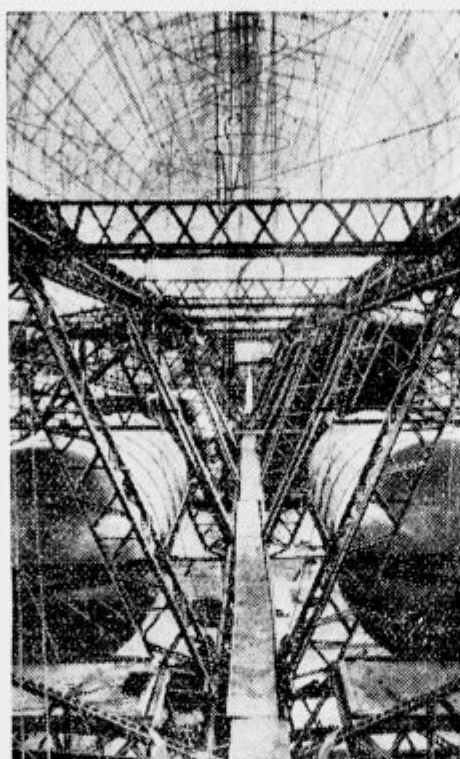
Notranjost nove zračne ladje — »Zeppelina«: hodnik in posode za olje.
