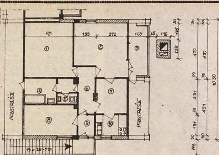
TLORIS STANOVANJA ST. 3 V PSO ŠENTJERNEJ M 1:100
