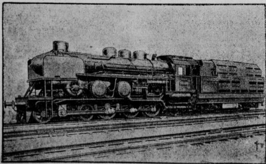
Nova Kruppova lokomotiva na turbine, ki vozi na progi Hannover—Köln. Doseže hitrost 110 km na uro. Namesto dosedaj običajnih parnih cilindrov ima dve parni turbini. Tender služi za ohlajevalne naprave, ki izpreminjajo iz turbine prihajajočo paro zopet v vodo.
