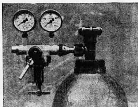
REDUCNI VENTIL »AGA-RUŠE« Z NAVZDOL OBRNjenIM REGULIRNIM VIJAKOM.
