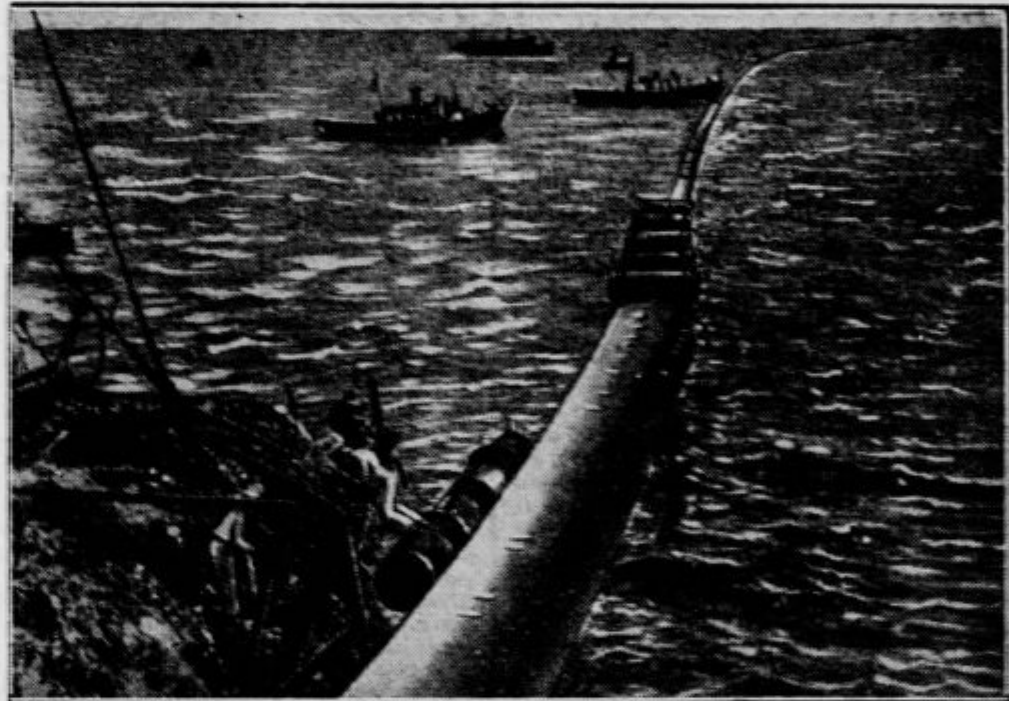
Izrada morske vodne sile. Francoski fizik Georges Claude je, kakor smo že poročali, napravil načrt, po katerem bi s pomočjo 2000 m dolge in 1,60 m močne jeklene cevi znatne razlike vodne temperature na površini (30°) in v globlini (5°) v zalivu Mantanza (Kuba) izkoristil za pridobivanje vodne sile. Pri tozadevnih delih so sedaj napravili velik korak naprej. Glavna težkoča je bila potopitev cevi, kar se je po dvakratnih ponesrečenih poskusih sedaj končno posrečilo.
