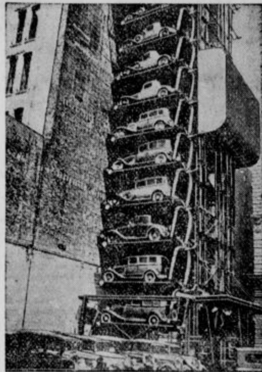
Garaža za avtomobile v nadstropjih. — Ameriški nebotičniki morajo imeti tudi velikanske garaže. Zato so v Chicagu napravili posebno garažo v nadstropjih, kamor dvigajo avtomobile s posebnimi dvigali, ki so podobna, recimo, dvigalu v Ljubljanskem dvoru, ki teče neprestano.
