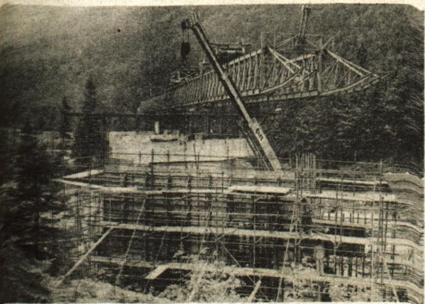
Ingradnja viadukta pod Belim poljem — Prek šestdeset delavcev temeljne organizacije Gradisa z Jesenic gradi od konca februarja pri Hručici viadukt, ki bo povezoval novo gorenjsko avtomobilsko cesto onkraj Save s karavanskim predorom. Zdaj so narejeni že štirje od skupno šestih opornikov viadukta, dva pa še gradijo. Viadukt, ki ga bodo zgradili predvidoma do konca septembra letos, bo dolg okrog 160 metrov in širok okrog 16 metrov. (Besedilo in slika: S. Saje)
